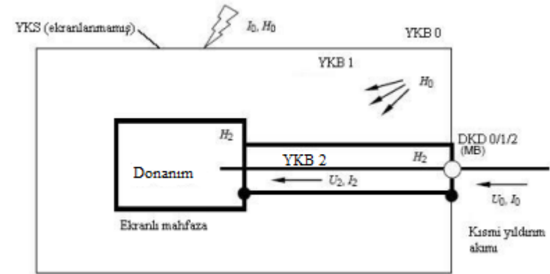
Şekil 7.5c- – YKB 1 girişinde DKD koruması yapılan ve iç hatları ekranlanan YEKS – Donanım, iletilen darbelere karşı korunmuştur ( U_2 \ll U_0 ve I_2 \ll I_0 ) ve ısınımla yayılan manyetik alanlara karşı da korunmuştur ( H_2 \ll H_0 )
